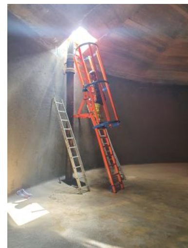
Échelle sécurisée au réservoir de la Folte à Cérilly
